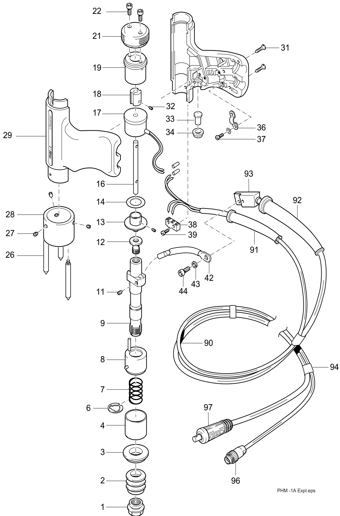
Abb. 8 - 3 Ersatzteile für Schweißpistole, Explosionszeichnung PHM-1A
